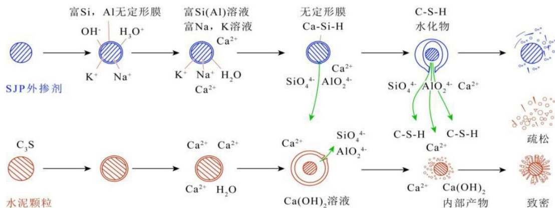
图1 水泥—聚合物溶剂化膜协调二次水化概念模型
