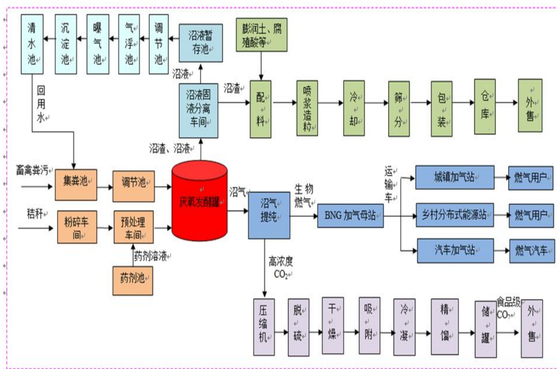
系统工艺流程图见图1。
