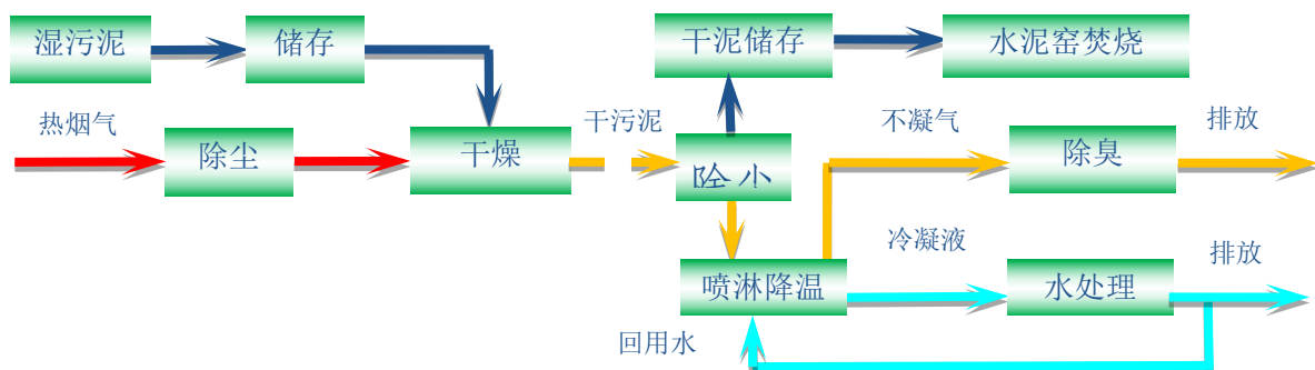
图2 污泥直接干化工艺
