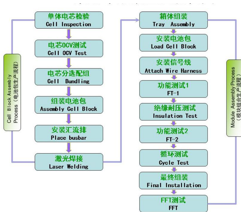
图2 电池组生产工艺流程示意图
